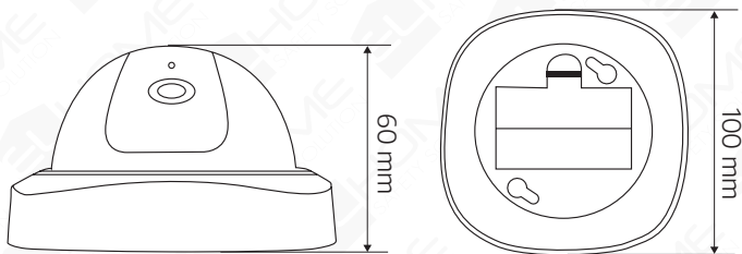
Rys. 2. Wymiary zewnętrzne atrapy AK-09B3
